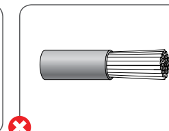
Жилы слишком выпрямлены
